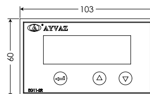
EG-11 2R Размеры панели управления
